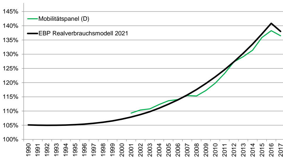
Abbildung 4. Gegenüberstellung EBP-Realverbrauchsmodell 2021 mit Flottenmesswerten von privat genutzten Autos (Daten aus ICCT 2019).
