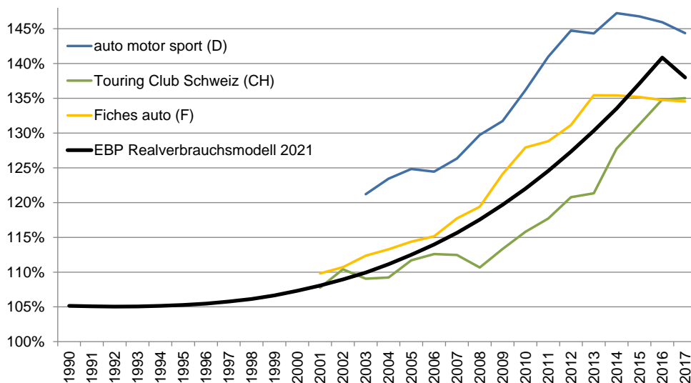
Abbildung 5. Gegenüberstellung EBP-Realverbrauchsmodell 2021 mit Daten aus Testfahrten von Automobilmagazinen (Daten aus ICCT 2019).
